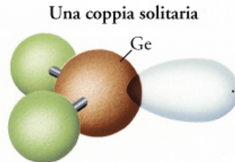
Angolare (GeCl 2 )
