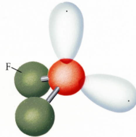
Angolare ( \text{OF}_2 )
