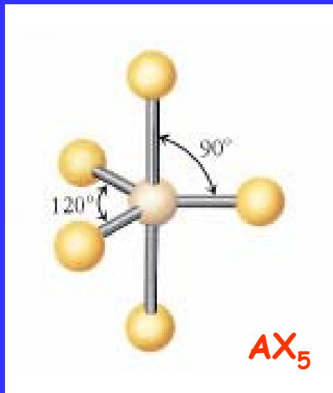
Trigonale bipiramidale
