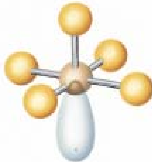
Piramidale quadrata
