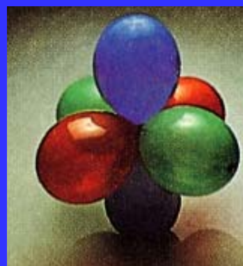
Ottaedrica
