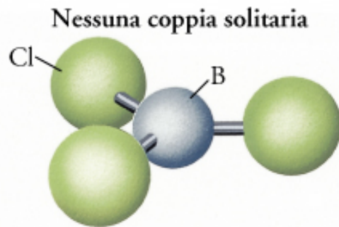
Planare triangolare (BCl 3 )
